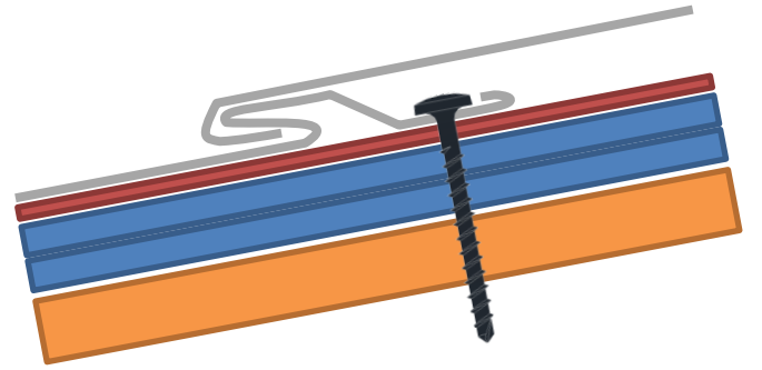
— 新設金属屋根 — ルーフィング — 既設スレート瓦 — 野地板
